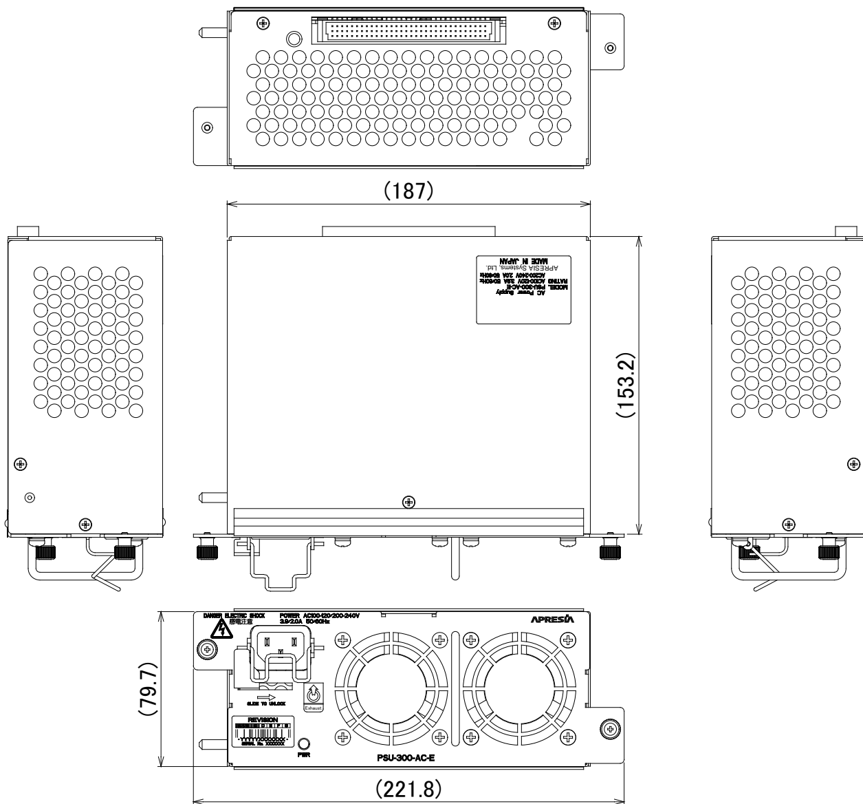
図 9-1 PSU-300-AC-E 外観図
