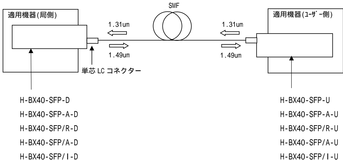
図 6-1 接続構成図
