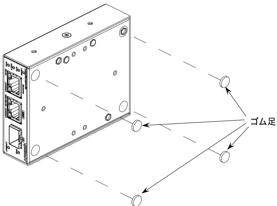
図 3-1 ゴム足の取り付け方法
