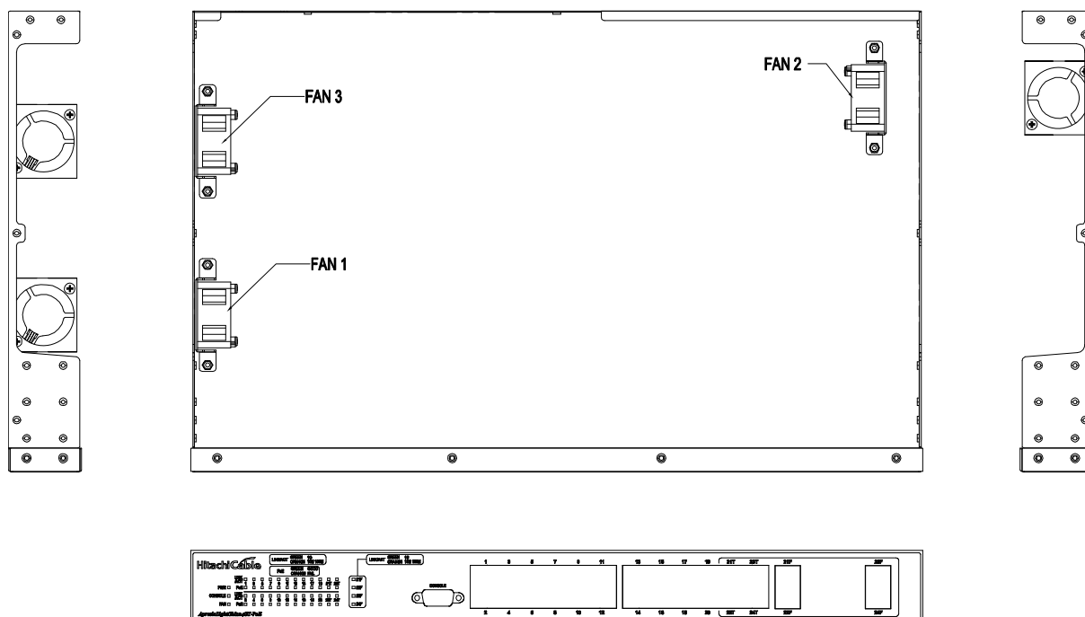
図 3-1 APLGM124GT-POE の FAN 位置図
