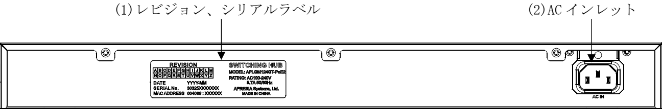
図 2-46 ApresiaLightGM124GT-PoE/PoE2 のリアパネル
