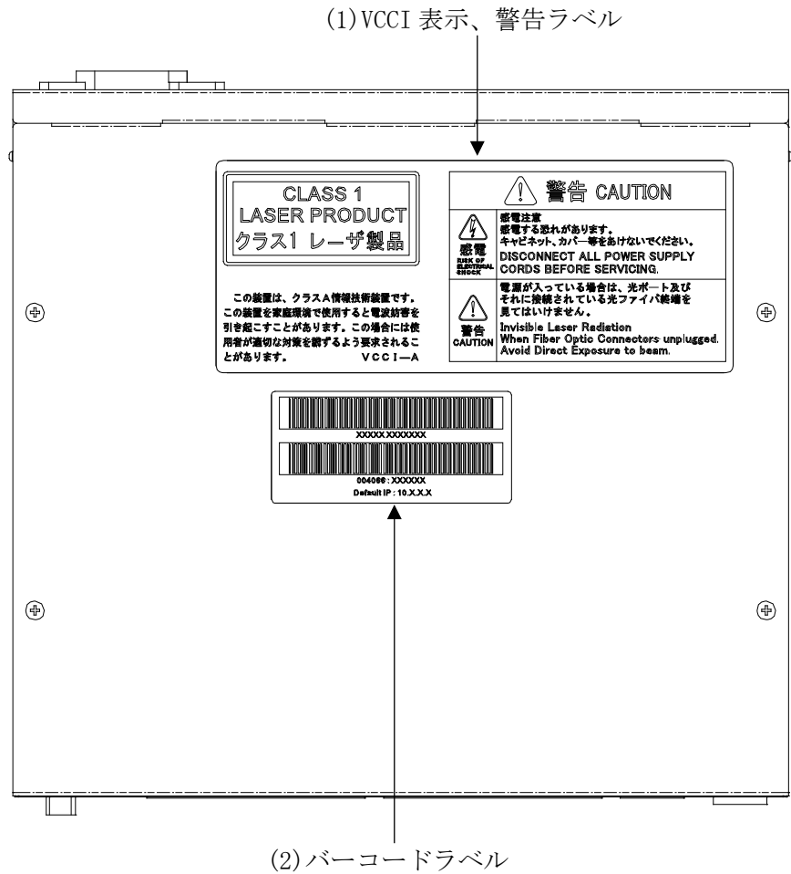
図 2-31 ApresiaLightGM118GT-SS のトップパネル
