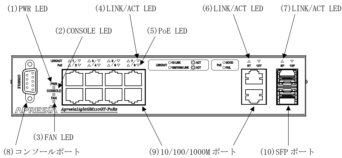
図 2-37 ApresiaLightGM110GT-PoE/PoE2 のフロントパネル
