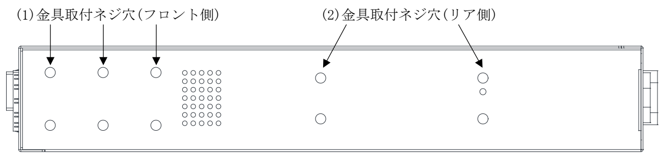
図 2-24 ApresiaLightFM116GT-PoE のサイドパネル
