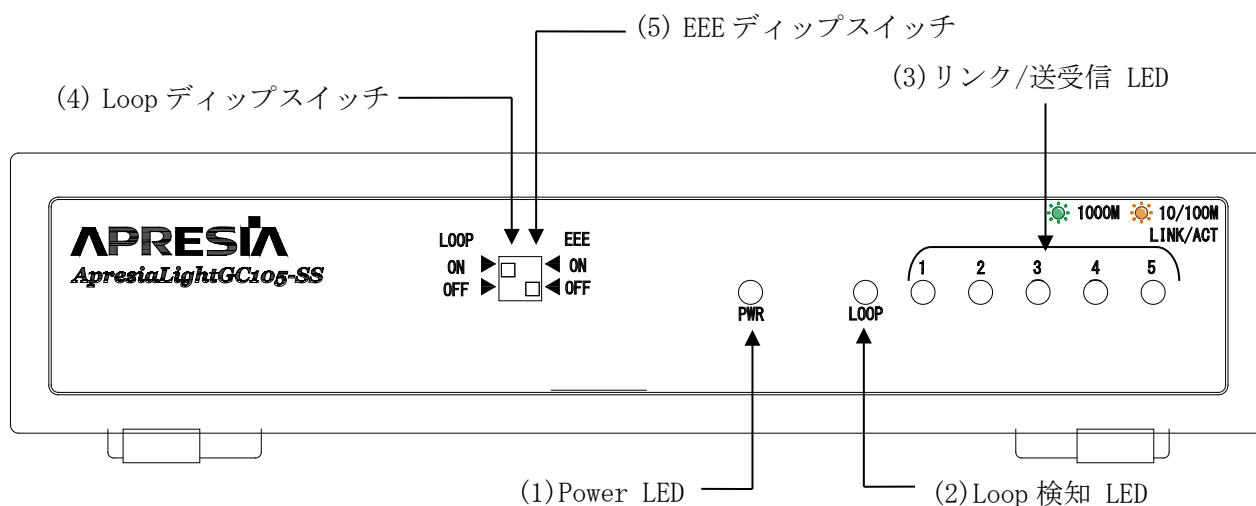
図 2-1 ApresiaLightGC105-SS のフロントパネルの構成
