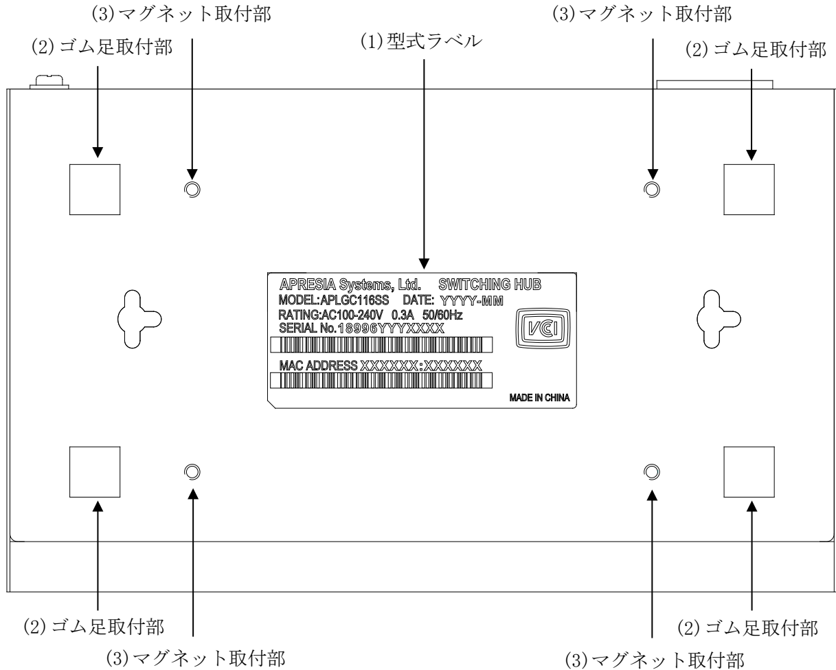
図 2-9 ApresiaLightGC116-SS のボトムパネルの構成
