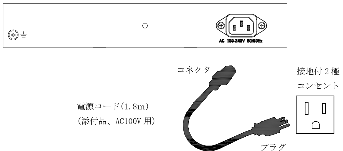
図 3-6 AC 電源の接続方法 (ApresiaLightGC124-SS の例)
