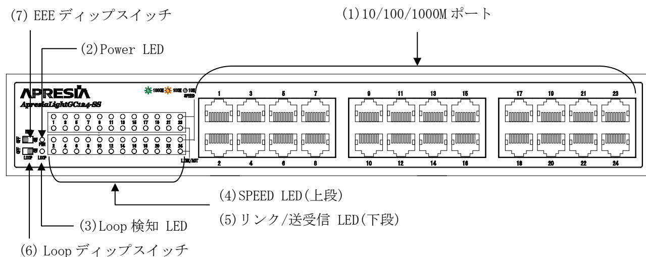
図 2-10 ApresiaLightGC124-SS のフロントパネルの構成
