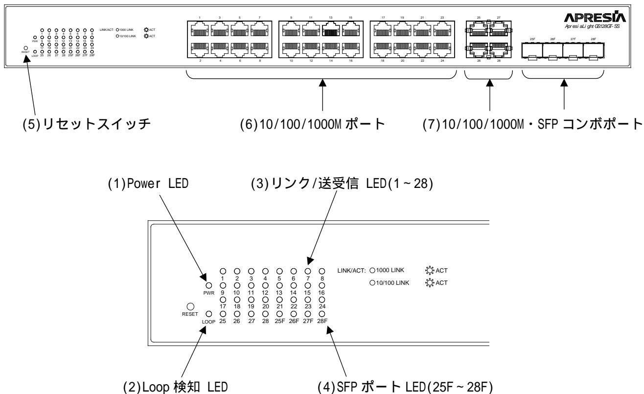
図 2-9 ApresiaLightGS128GT-SS のフロントパネルの構成
