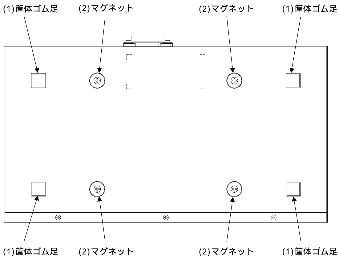
図 2-19 ApresiaLightGS110GT-PoE のボトムパネルの構成
