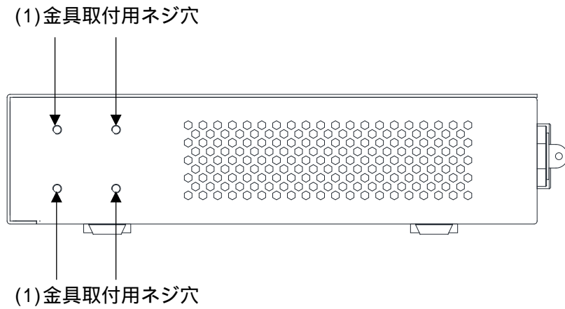
図 2-8 ApresiaLightGS120GT-SS のサイドパネルの構成
