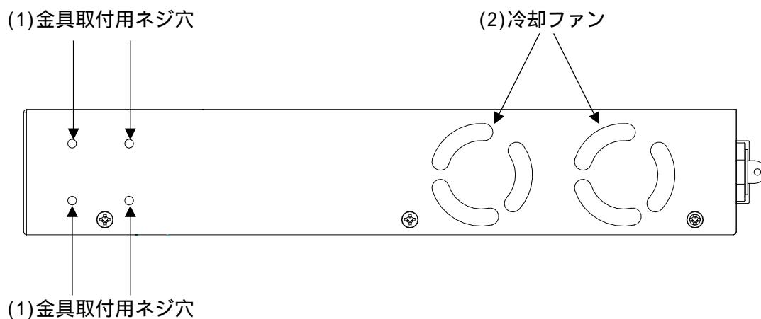
図 2-24 AprasiaLightGS120GT-PoE のサイドパネルの構成
