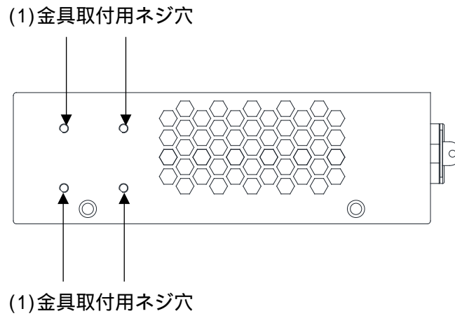
図 2-12 ApresiaLightGS128GT-SS のサイドパネルの構成
