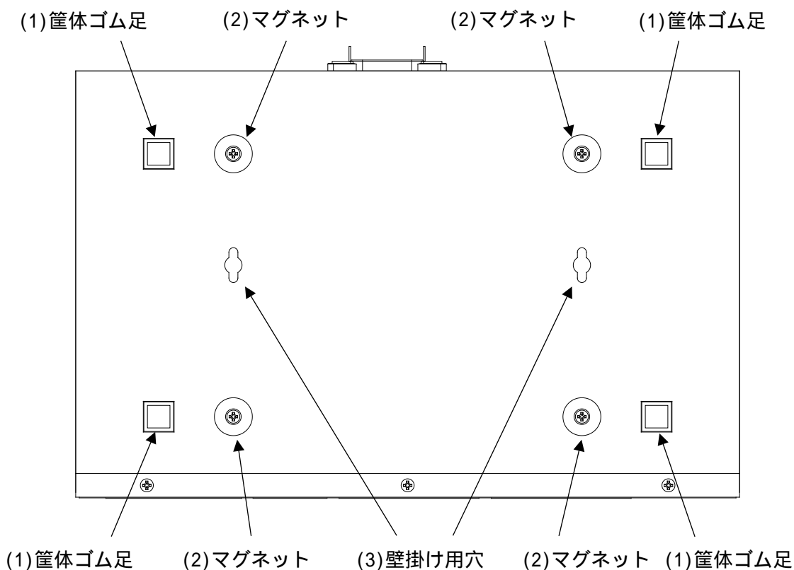
図 2-7 ApresiaLightGS120GT-SS のボトムパネルの構成
