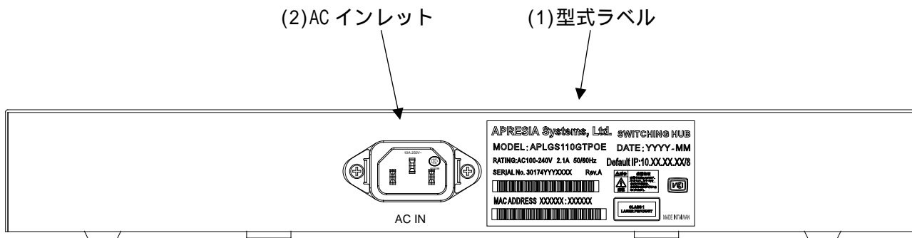
図 2-18 AprasiaLightGS110GT-PoE のリアパネルの構成
