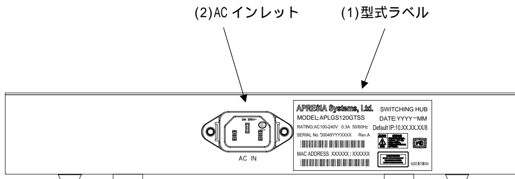
図 2-6 ApresiaLightGS120GT-SS のリアパネルの構成
