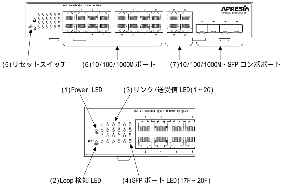
図 2-5 ApresiaLightGS120GT-SS のフロントパネルの構成
