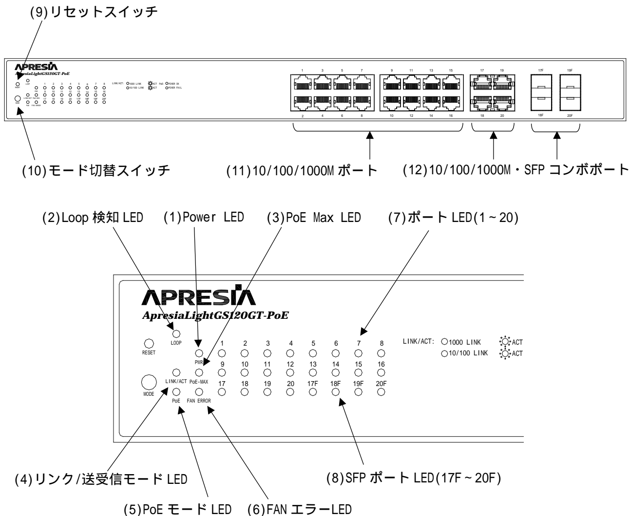
図 2-21 ApresiaLightGS120GT-PoE のフロントパネルの構成
