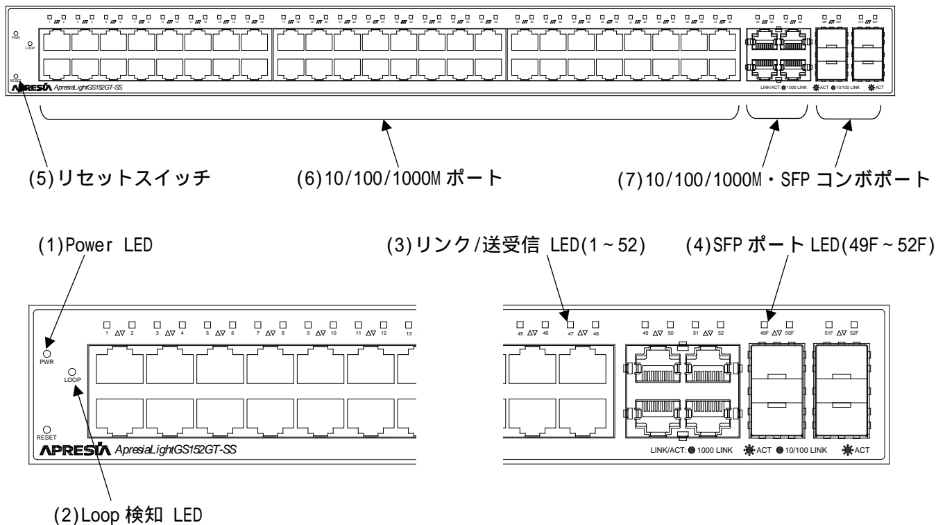
図 2-13 ApresiaLightGS152GT-SS のフロントパネルの構成
