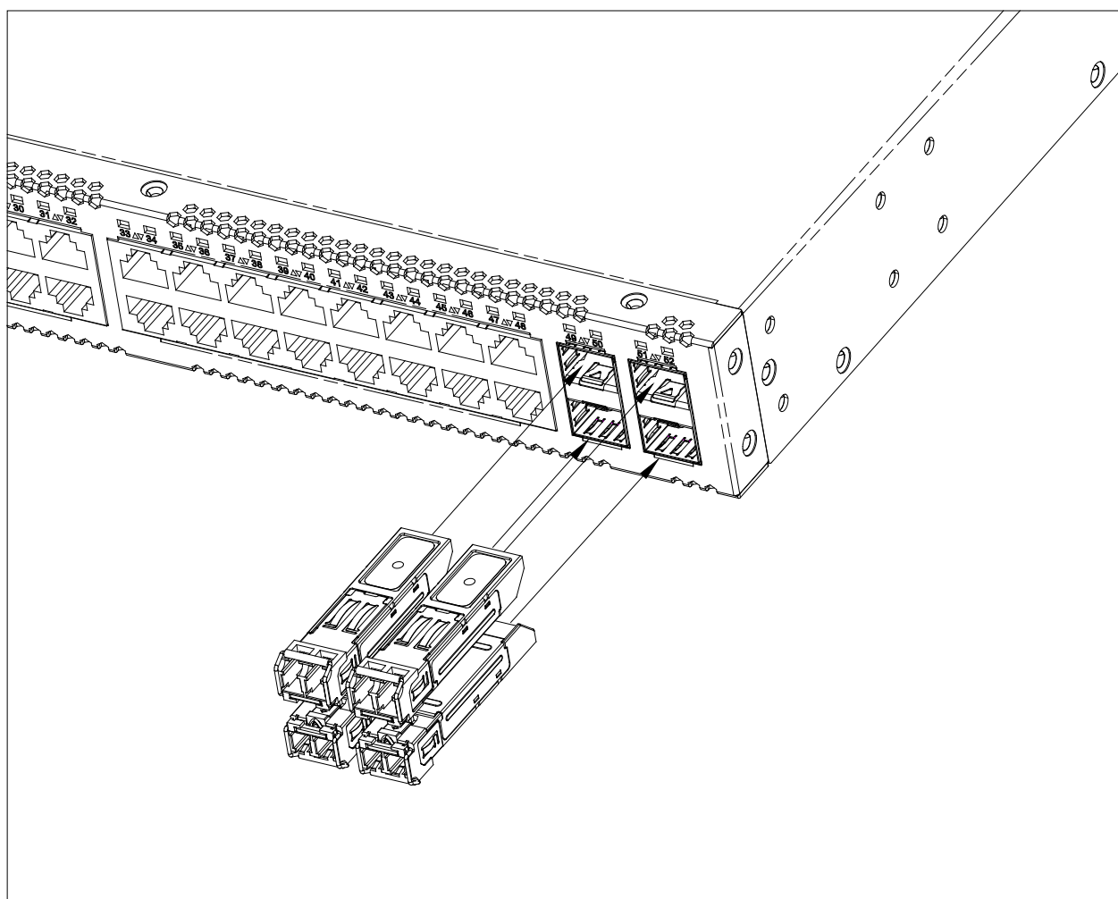
図 2-30 SFP の接続
