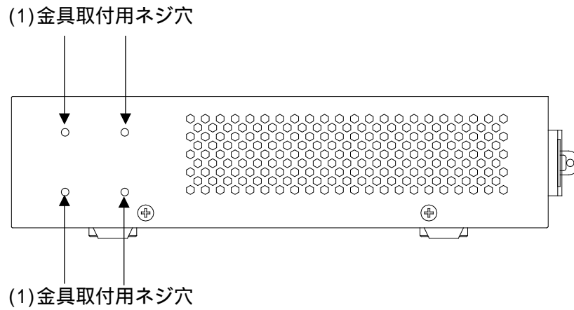
図 2-4 ApresiaLightGS110GT-SS のサイドパネルの構成
