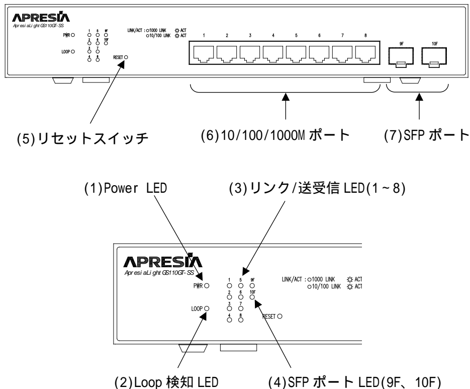
図 2-1 ApresiaLightGS110GT-SS のフロントパネルの構成
