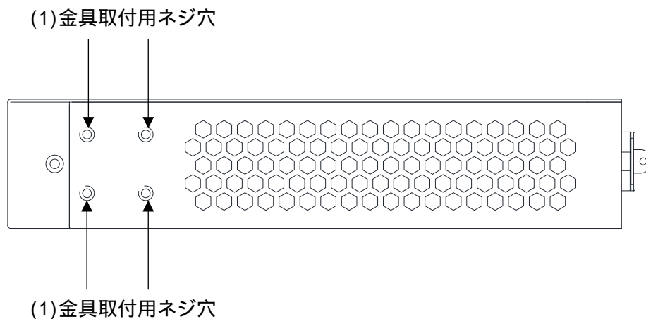
図 2-16 ApresiaLightGS152GT-SS のサイドパネルの構成
