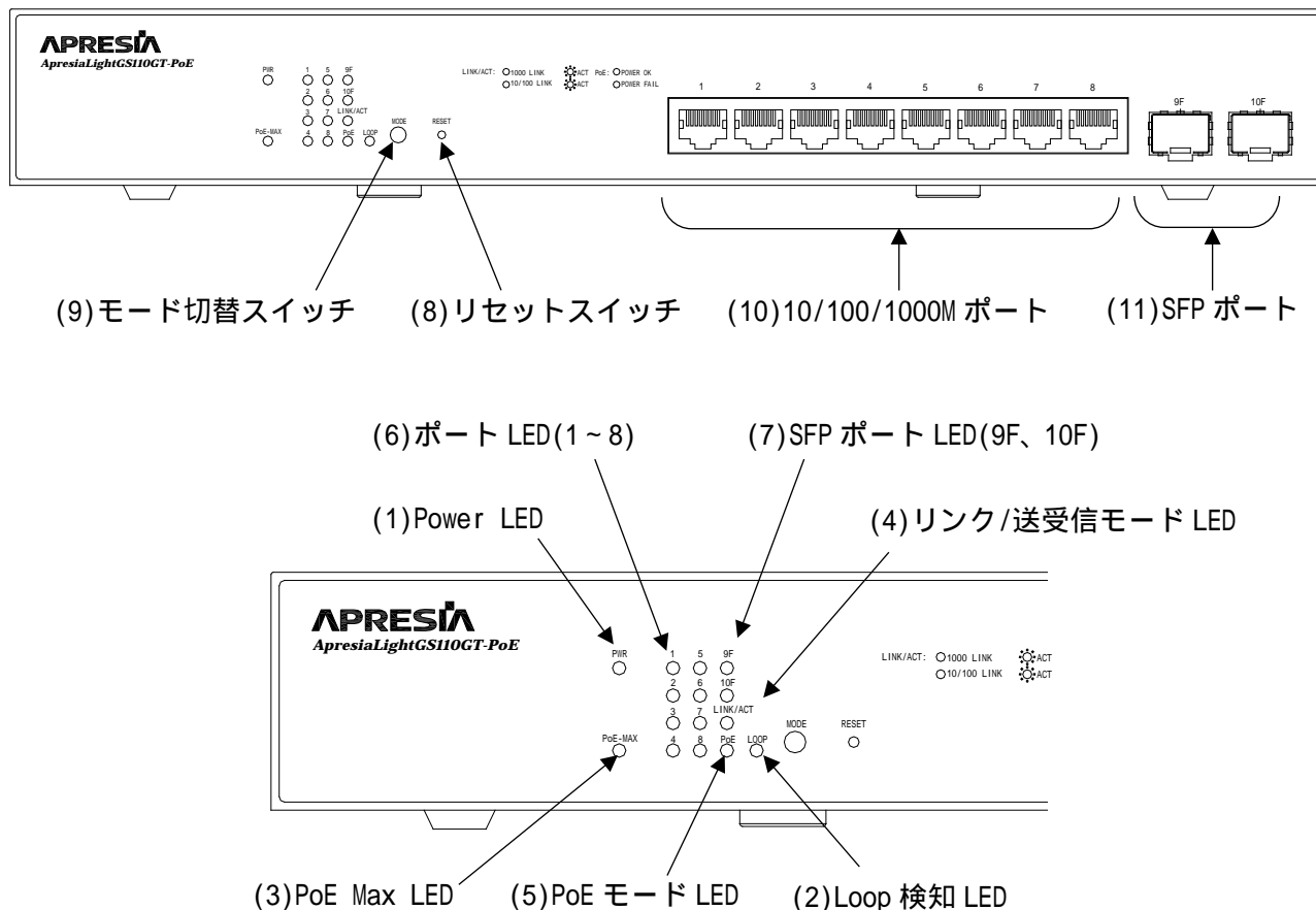
図 2-17 ApresiaLightGS110GT-PoE のフロントパネルの構成
