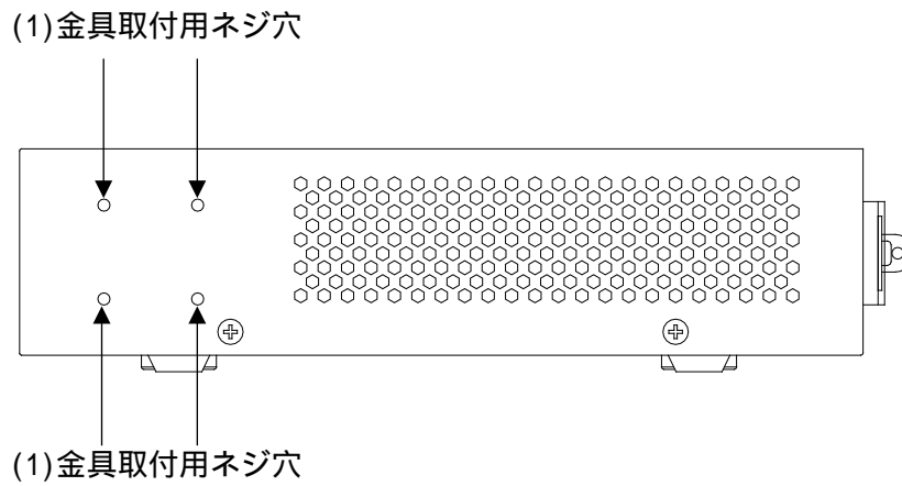
図 2-20 ApresiaLightGS110GT-PoE のサイドパネルの構成
