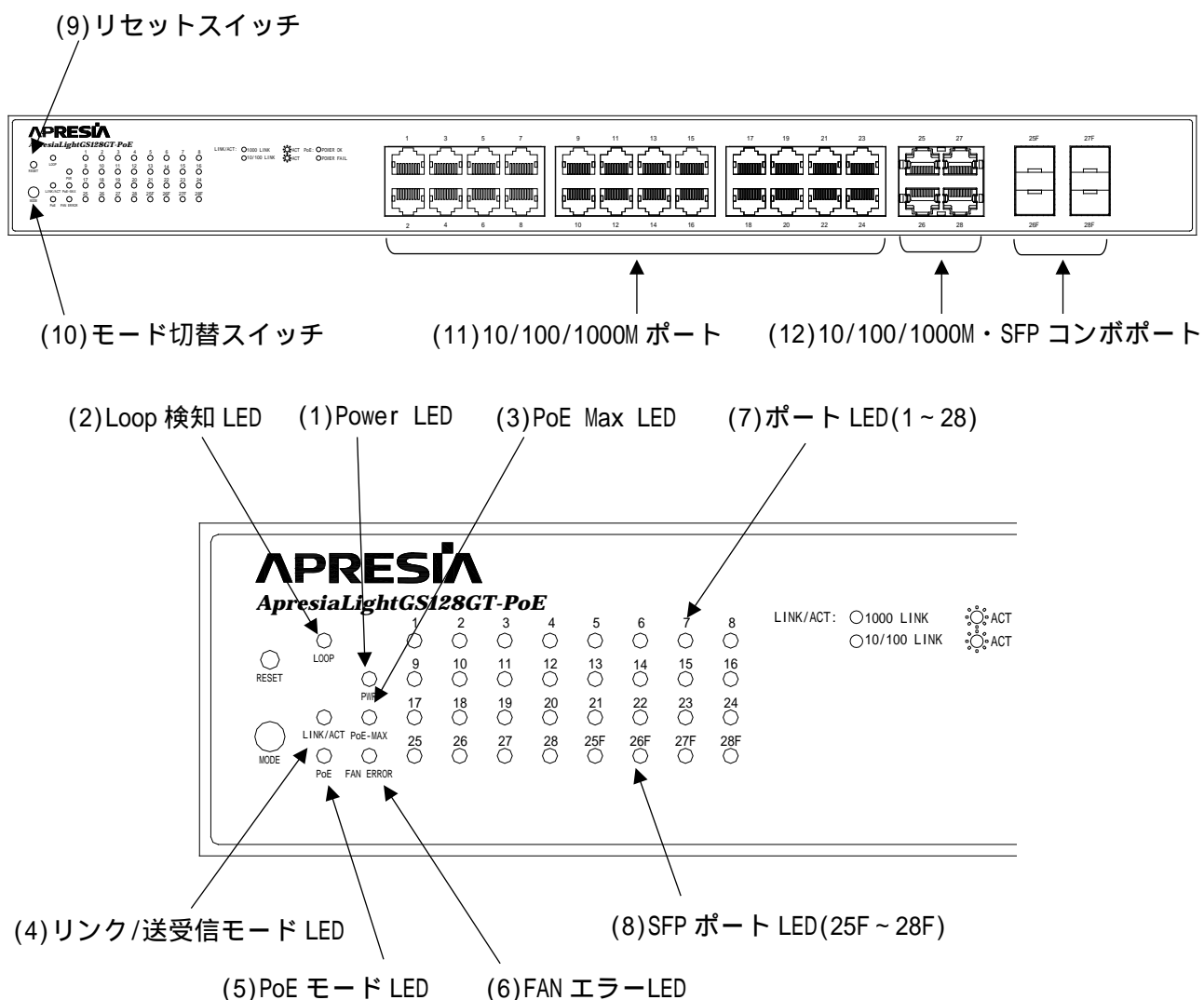
図 2-25 ApresiaLightGS128GT-PoE のフロントパネルの構成
