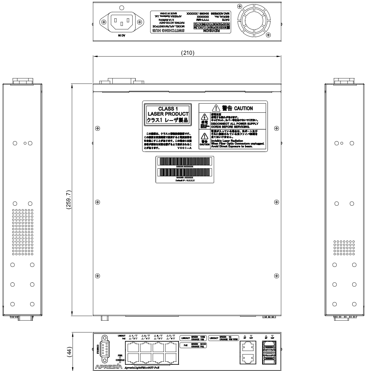
図 11-1 ApresiaLightFM108GT-PoE 外観図
