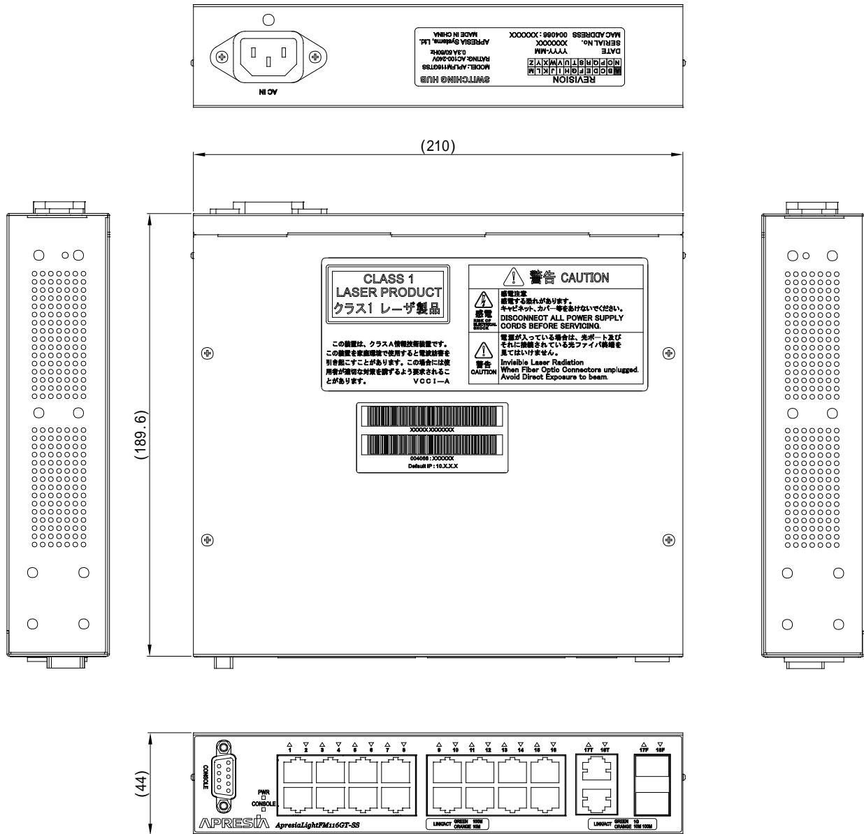
図 11-1 ApresiaLightFM16GT-SS 外観図
