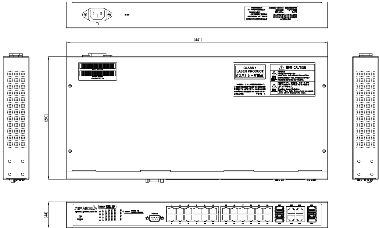
図 11-1 ApresiaLightFM124GT-SS 外観図
