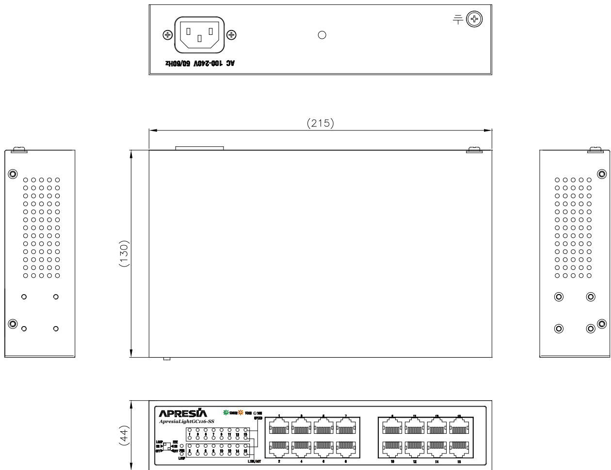
図 11-3 ApresiaLightGC116-SS 外観図
