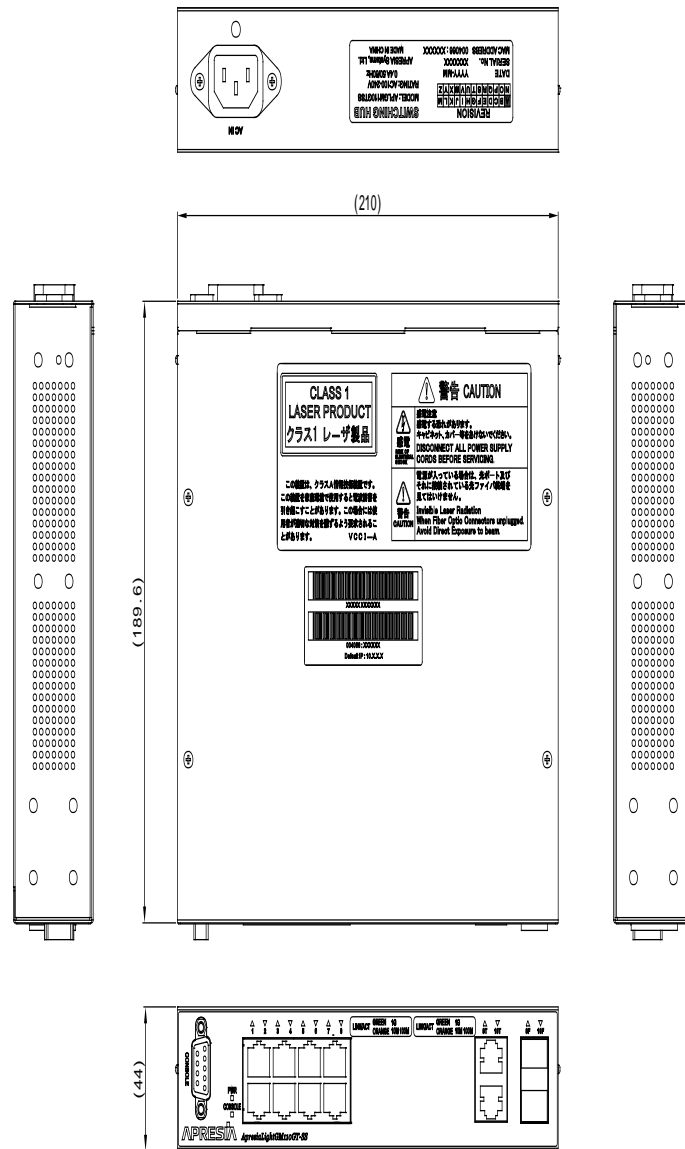
図 11-1 ApresiaLightGM110GT-SS 外観図
