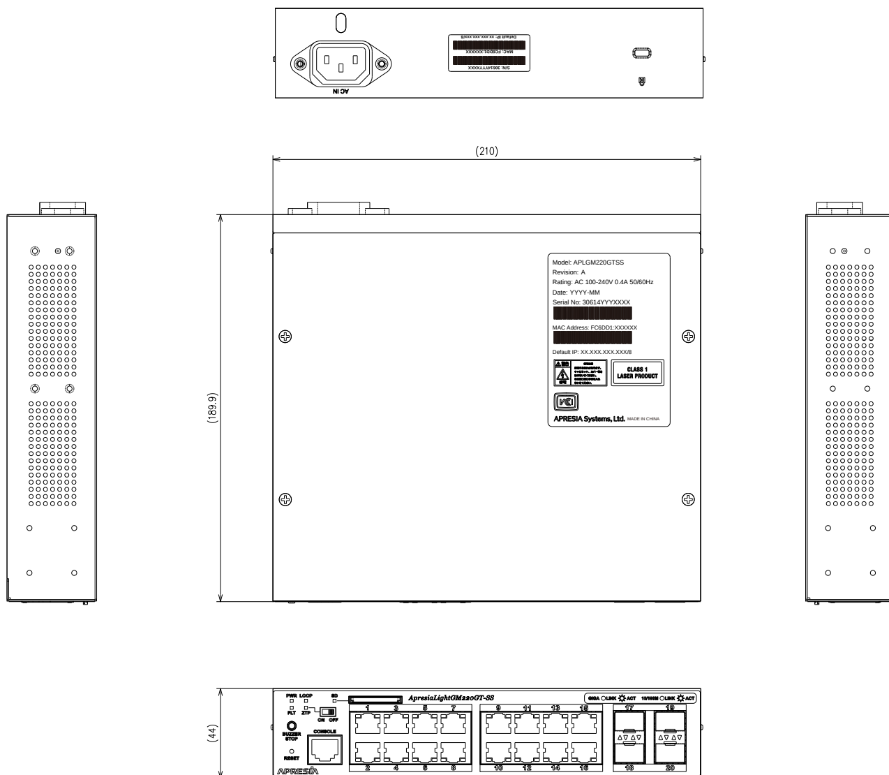
図 10-2 ApresiaLightGM220GT-SS 外観図
