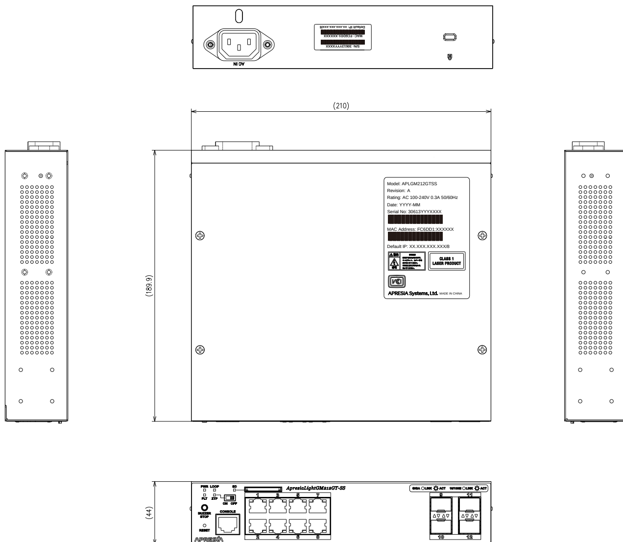
図 10-1 ApresiaLightGM212GT-SS 外観図
