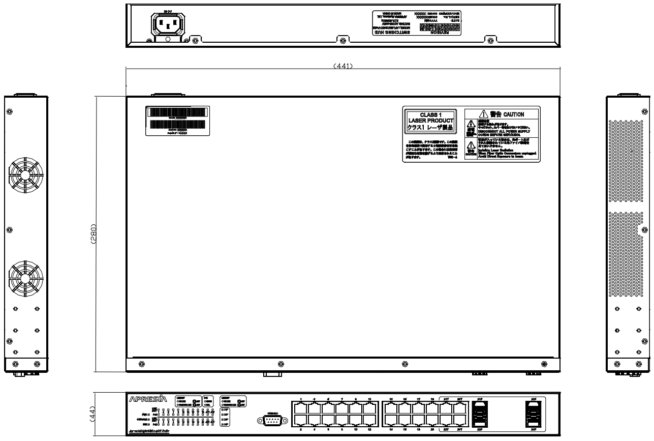
図 10-3 ApresiaLightGM124GT-PoE2 外観図
