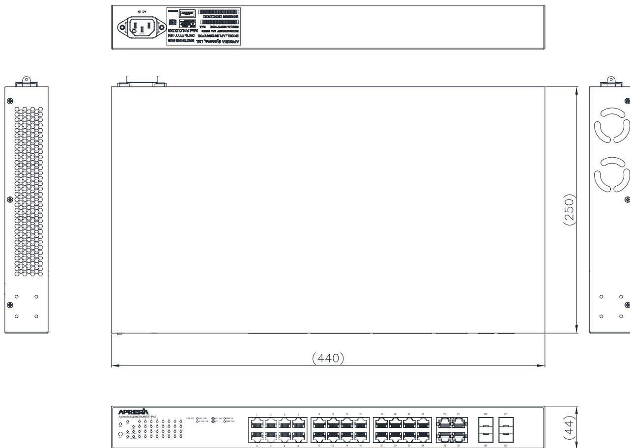
図 10-3 ApresiaLightGS128GT-PoE 外観図
