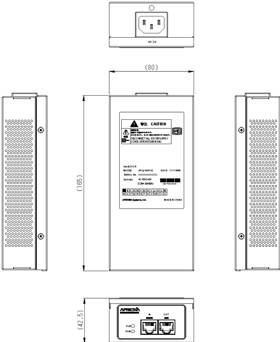
図 10-1 ApresiaLight IJ-1GPoE 外観図
