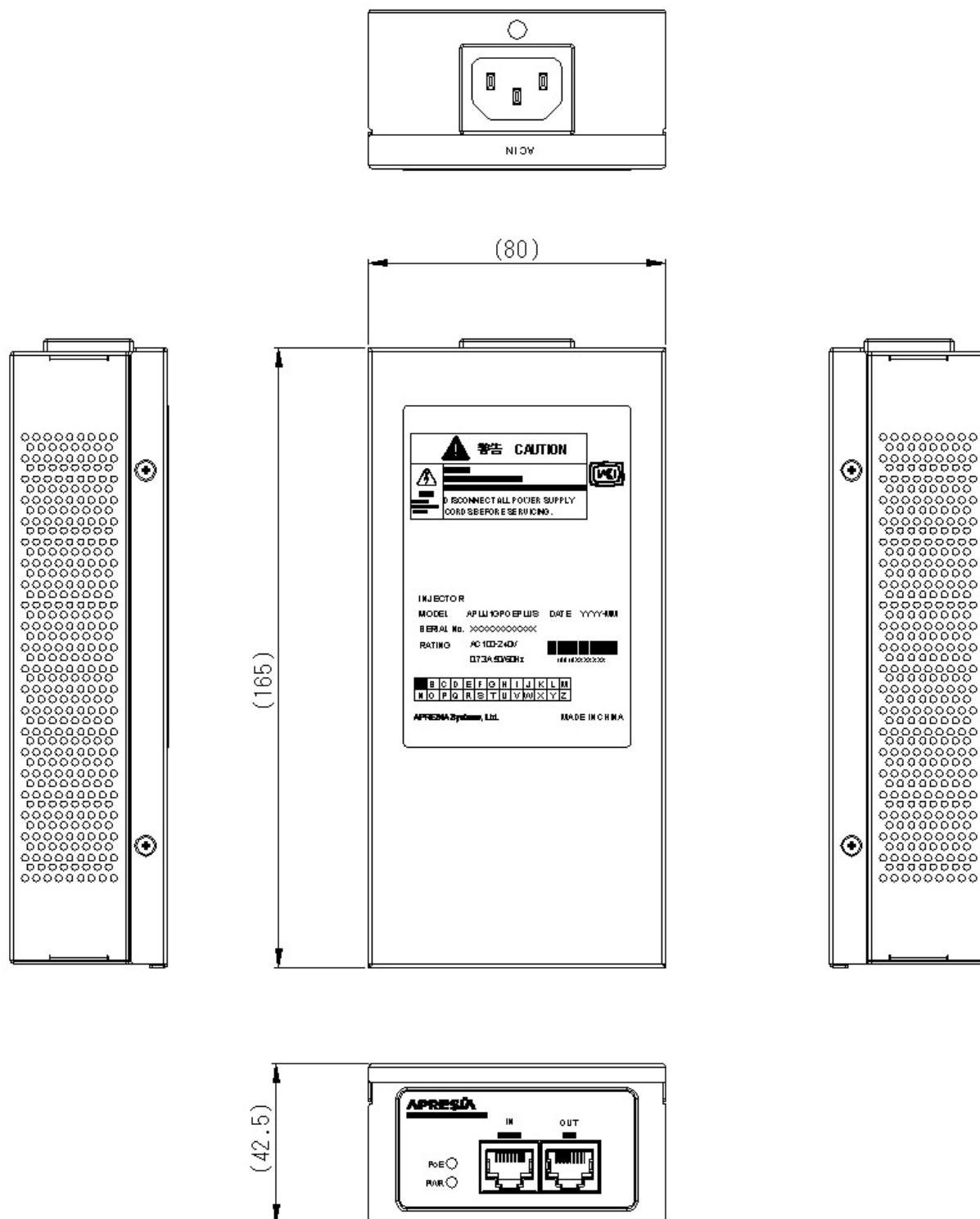
図 10-2 ApresiaLight IJ-1GPoE-Plus 外観図
